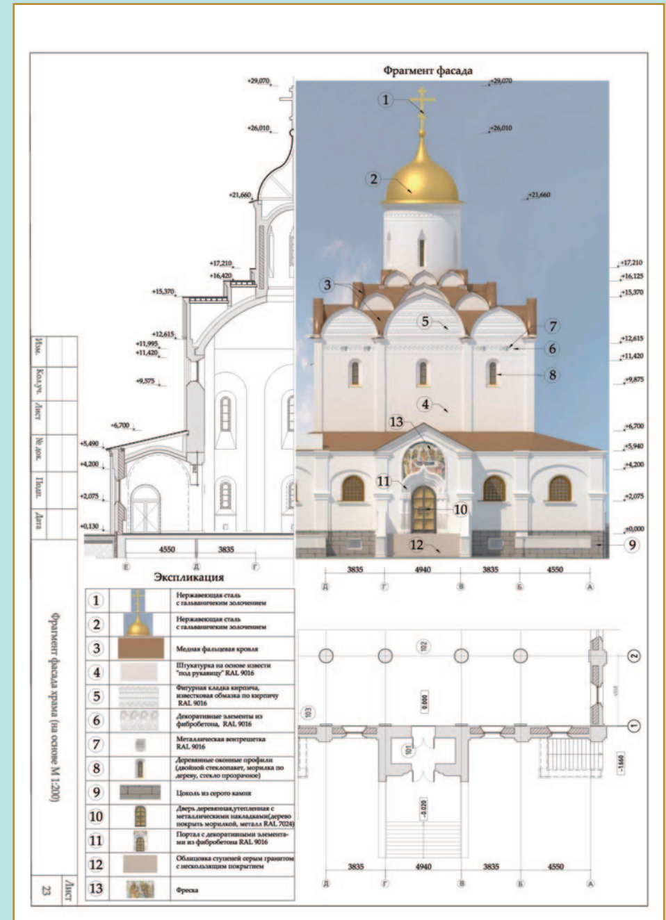
Проект храма. Западный фасад. Разрез
